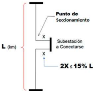
Figura 2.1 Longitud de la Derivación
