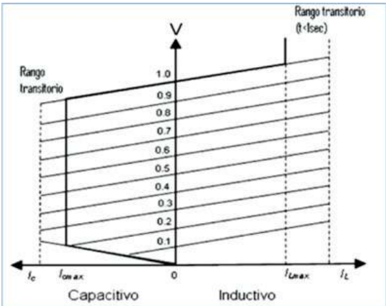
Figura 5.8. Curva característica V-I del STATCOM
