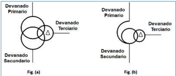
Figura 5.5. (a) Transformador, (b) Autotransformador
