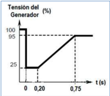
Figura 4.1. Hueco de tensión por falla trifásica en el SEIN, visto en bornes del generador
