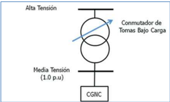
Figura 4.3. Transformador elevador con regulación bajo carga
