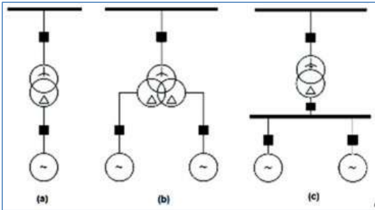
Figura 2.7 Configuraciones permitidas generador-transformador para CGC
